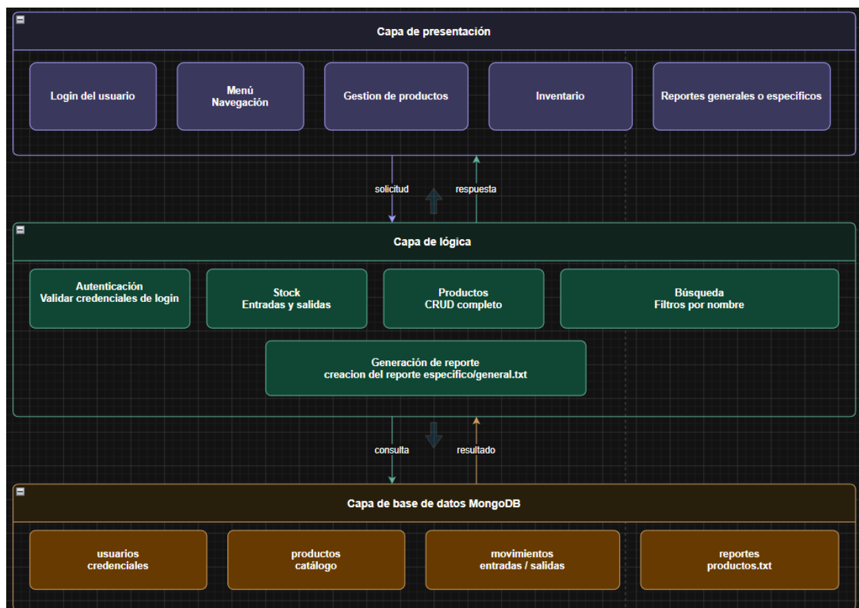
Figura 1. Diagrama de Capas del Sistema
