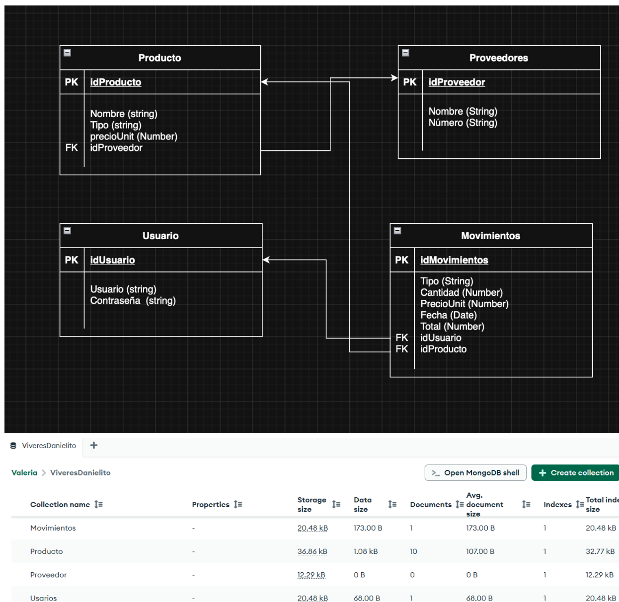
Figura 7. Diagrama Físico Base de Datos del Sistema
