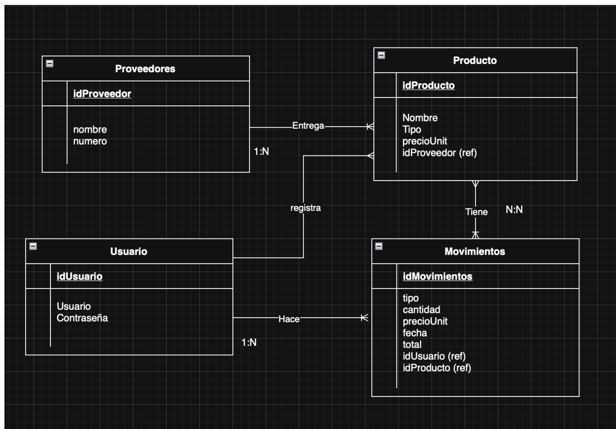
Figura 6. Diagrama Base de Datos del Sistema
