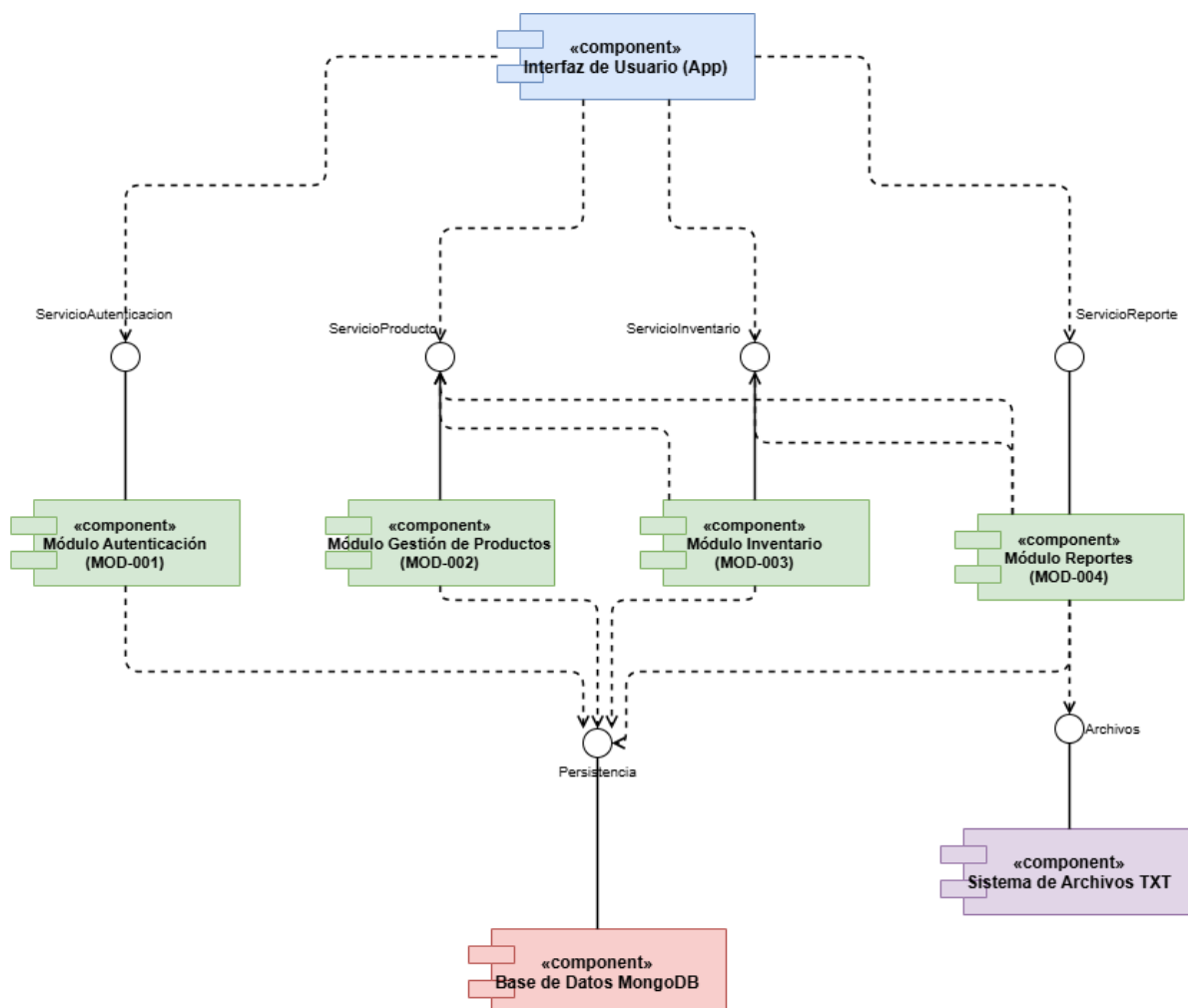
Figura 3. Diagrama de Componentes
